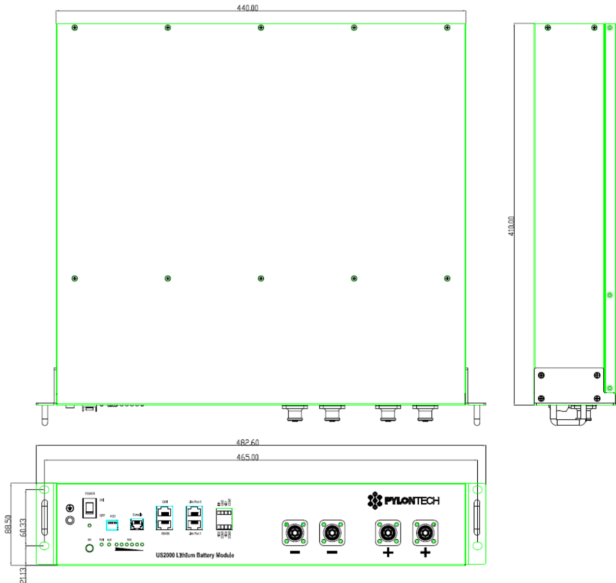
Abbildung 1: Dimensionen
